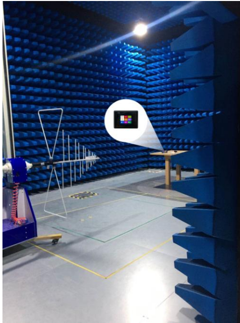
图 5-4 RE 测试图
