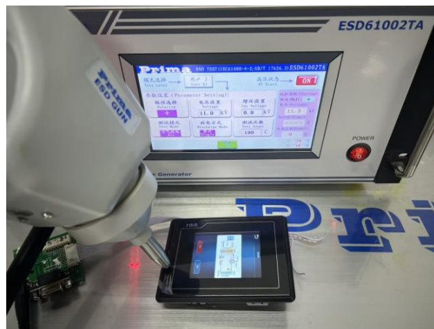
图 5-2 ESD 测试图
