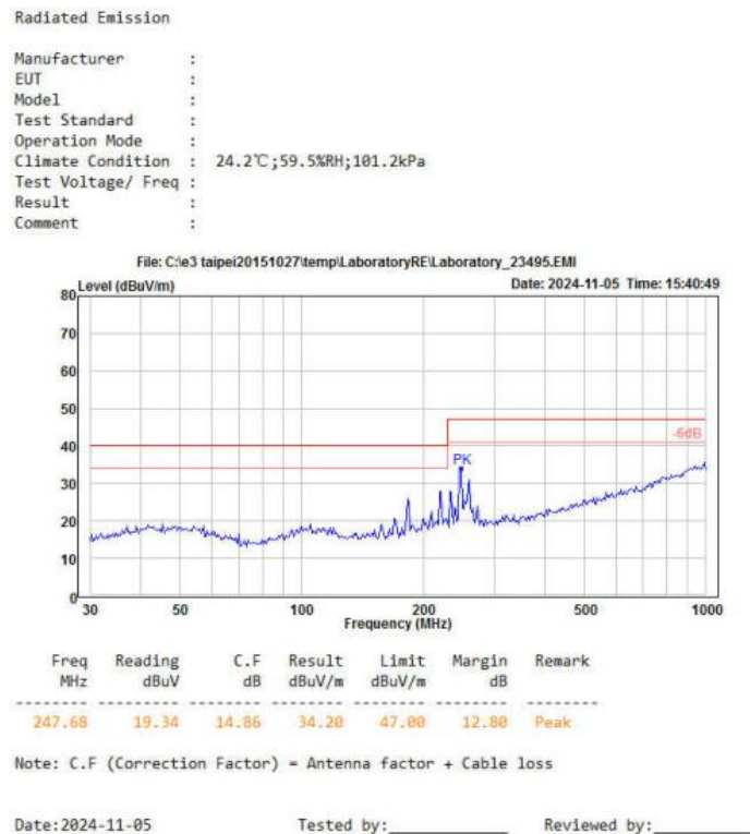
图 5-5 RE 测试水平方向
