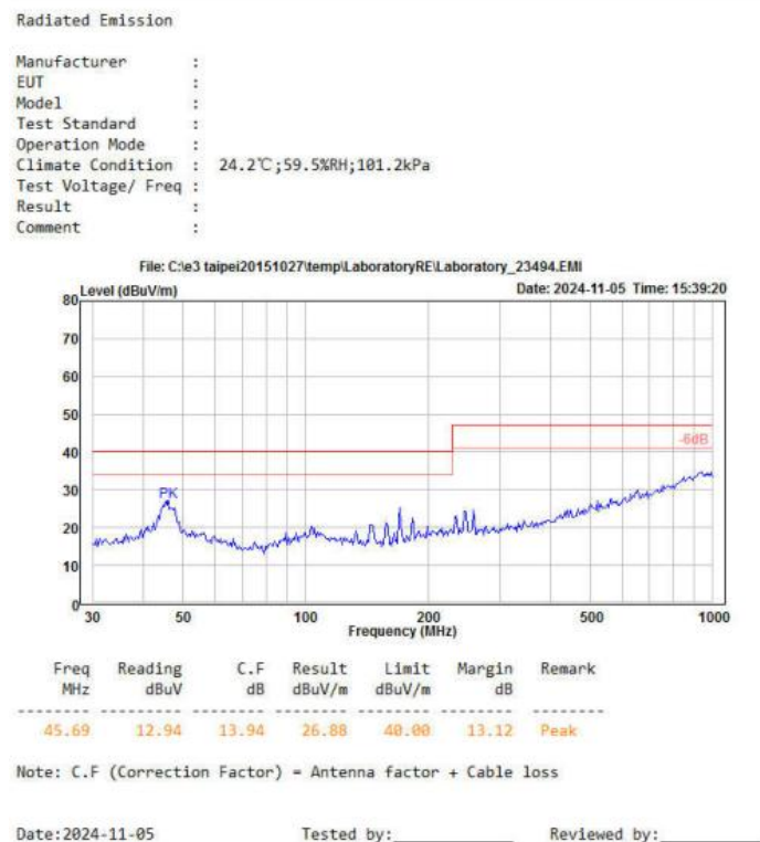
图 5-6 RE 测试垂直方向
